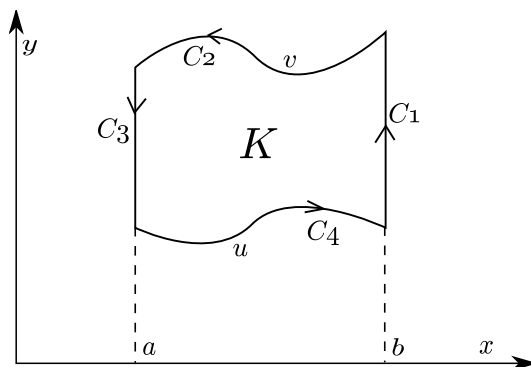
FIG. 2.3 – Représentation du compact K
