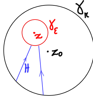
FIG. 3.3 – Le point z se trouve dans le cercle
