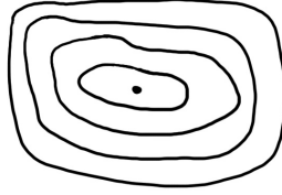
FIG. 2.6 – Homotopie de chemins fermés
