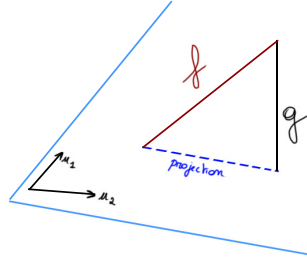
FIG. 4.1 – Projection orthogonale généralisée
