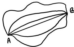
FIG. 2.5 – Homotopie de chemins à extrémités fixes
