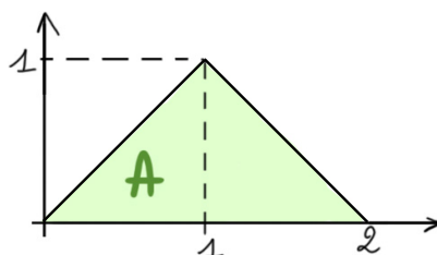
FIG. 1.1 – Représentation de l'ensemble A
