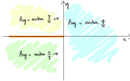
FIG. 3.1 – Valeur de l'argument dans le plan complexe
