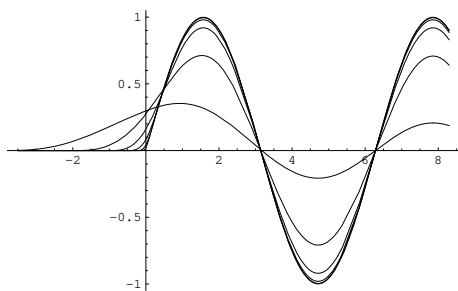
Convergence des solutions u_m de (1.1).
