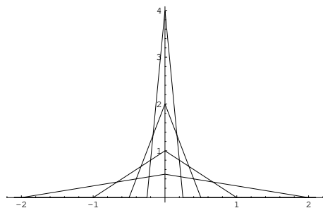
La suite de fonctions f_m .
