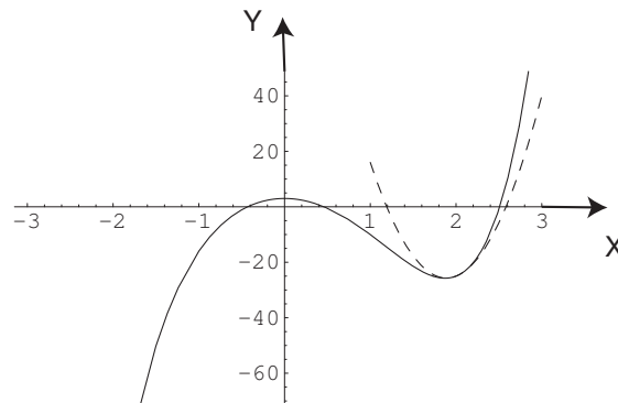
Graphique de f et de son approximation (en pointillés) à l'ordre 2 en x_0 = 2 (repère orthogonal non normé)
